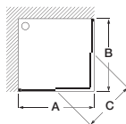
Victoria 2L2* para platos de ducha rectangulares
